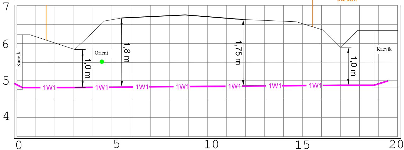
Ristmeväli RV-1 Riigitee nr 19340 Uulu-Laadi tee teemaal km 2,92 Ø110 19 m 1250N Kinnine läbindamine
